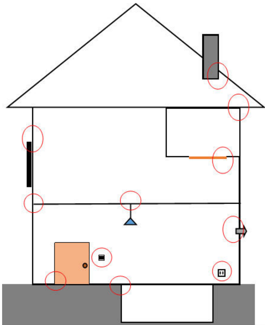
Principales sources d'arrivées d'air parasites dans un logement
