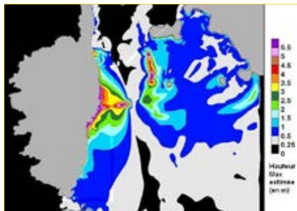
Source : BRGM - glissements gravitaires
