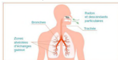
Voies atteintes par l'inhalation du radon et de ses descendants
