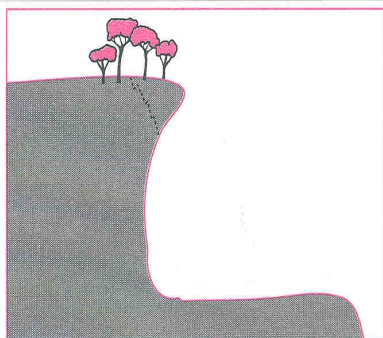
Fig. 1 : L'aléa
