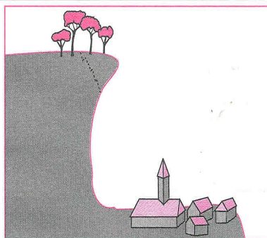
Fig. 2 : Les enjeux
