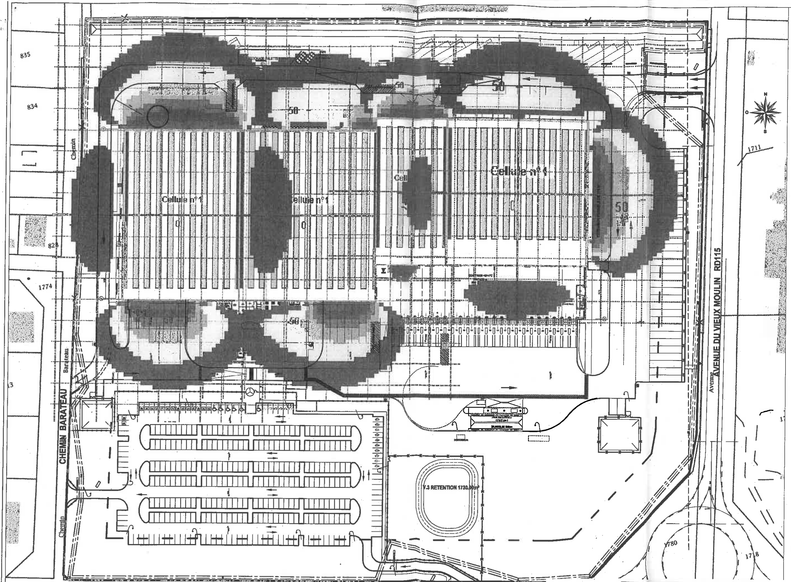
TRANSGOURMET - SAINT LOUBES - PLAN DES FLUX THERMIQUES GENERAL PORTER A CONNAISSANCE JUILLET 2017 - SANS ECHELLE
