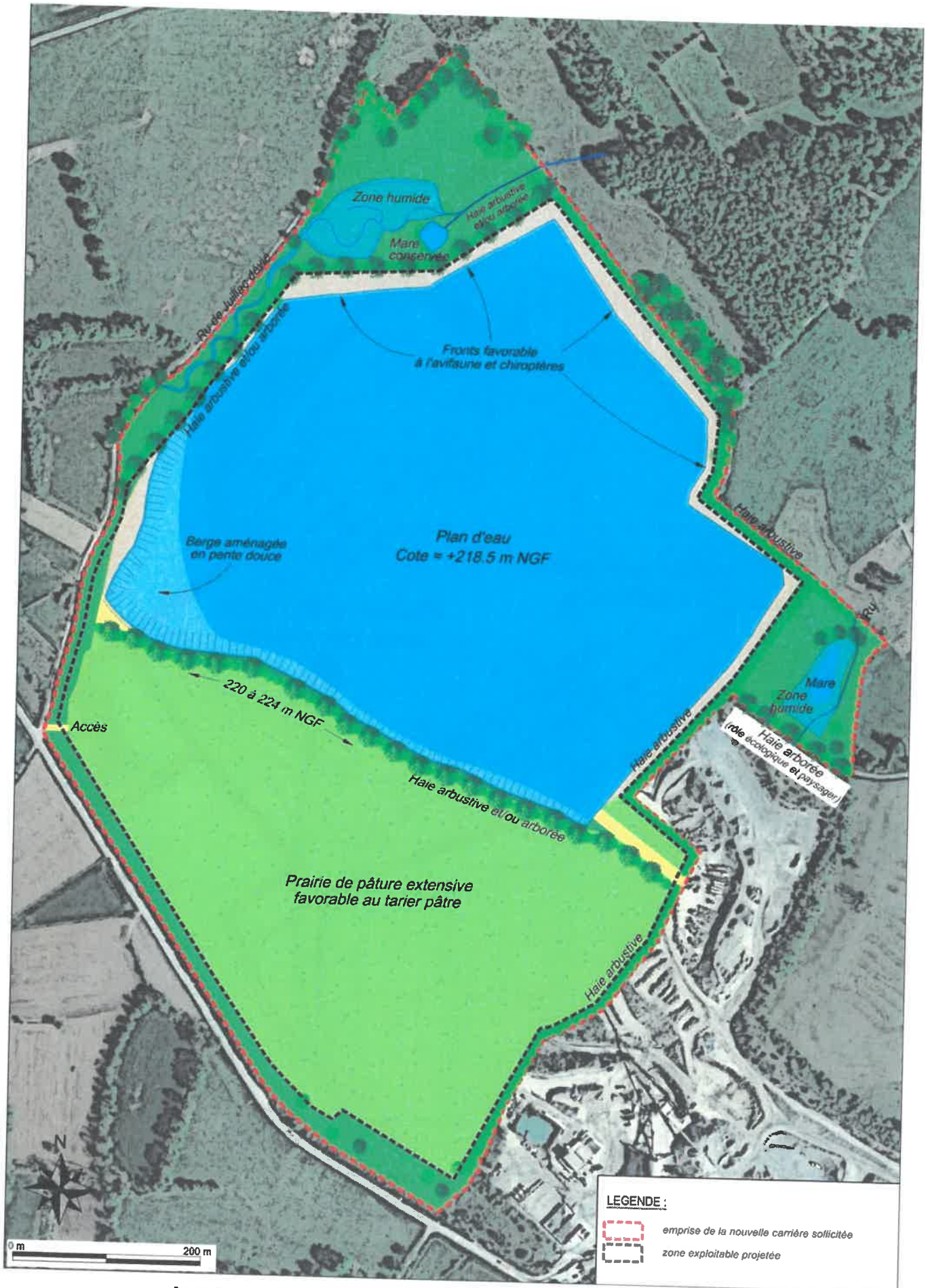
plan de remise en état à long terme après remontée des eaux
