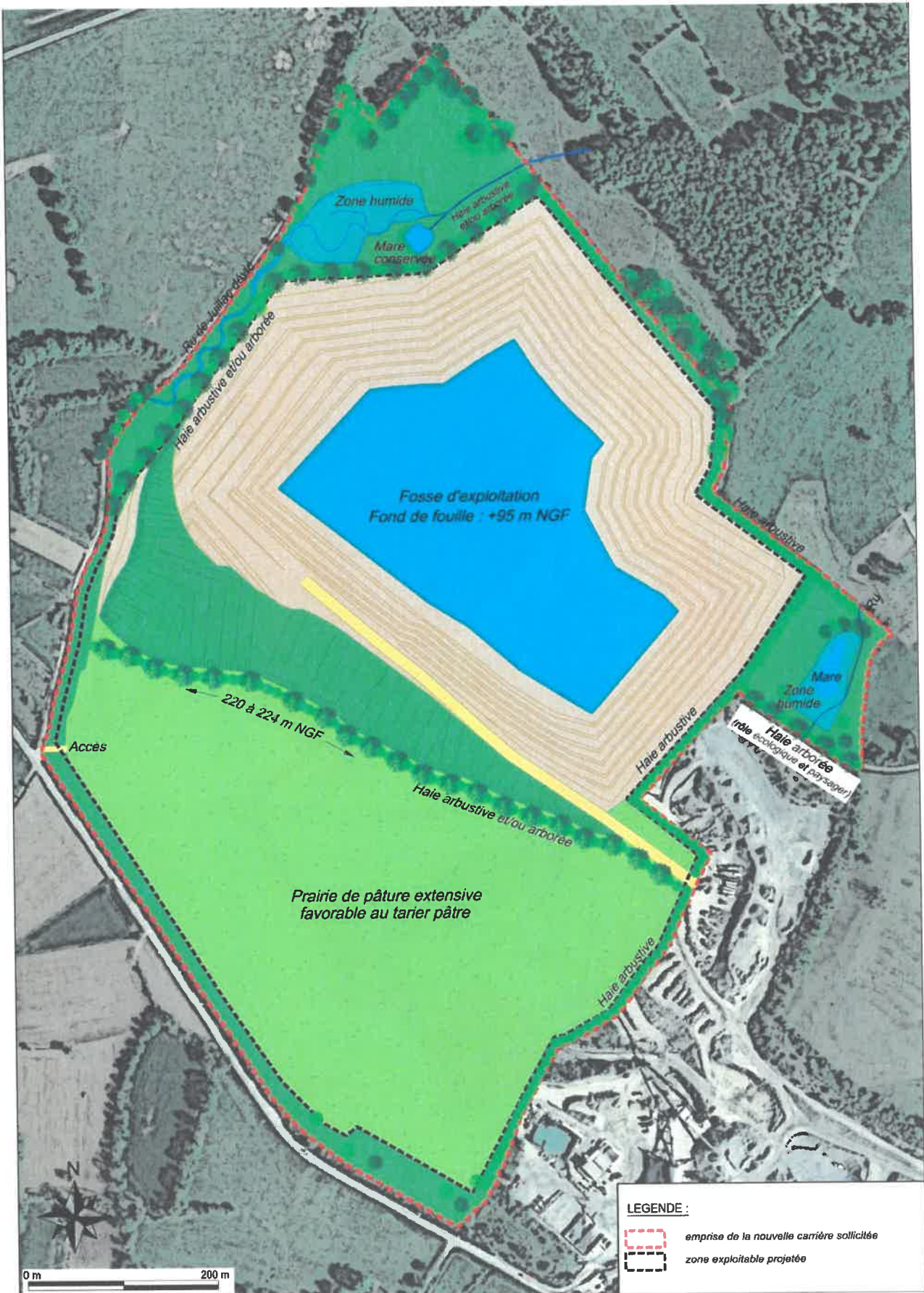
plan de remise en état en fin d'exploitation
