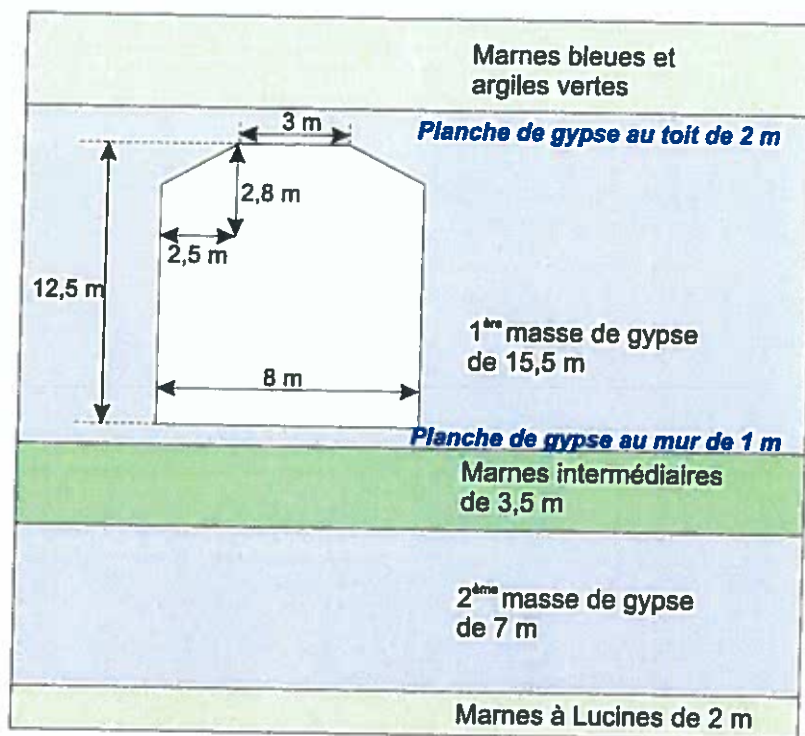
Géométrie des galeries (vue en coupe)
